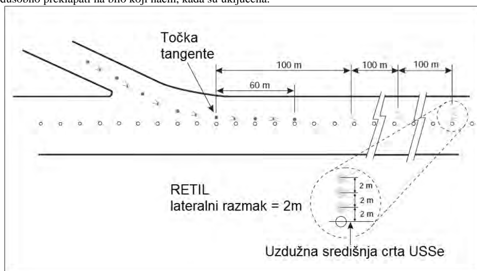
Slika 5-25. Svjetlosni pokazivači brzih izlaznih staza za vožnju
