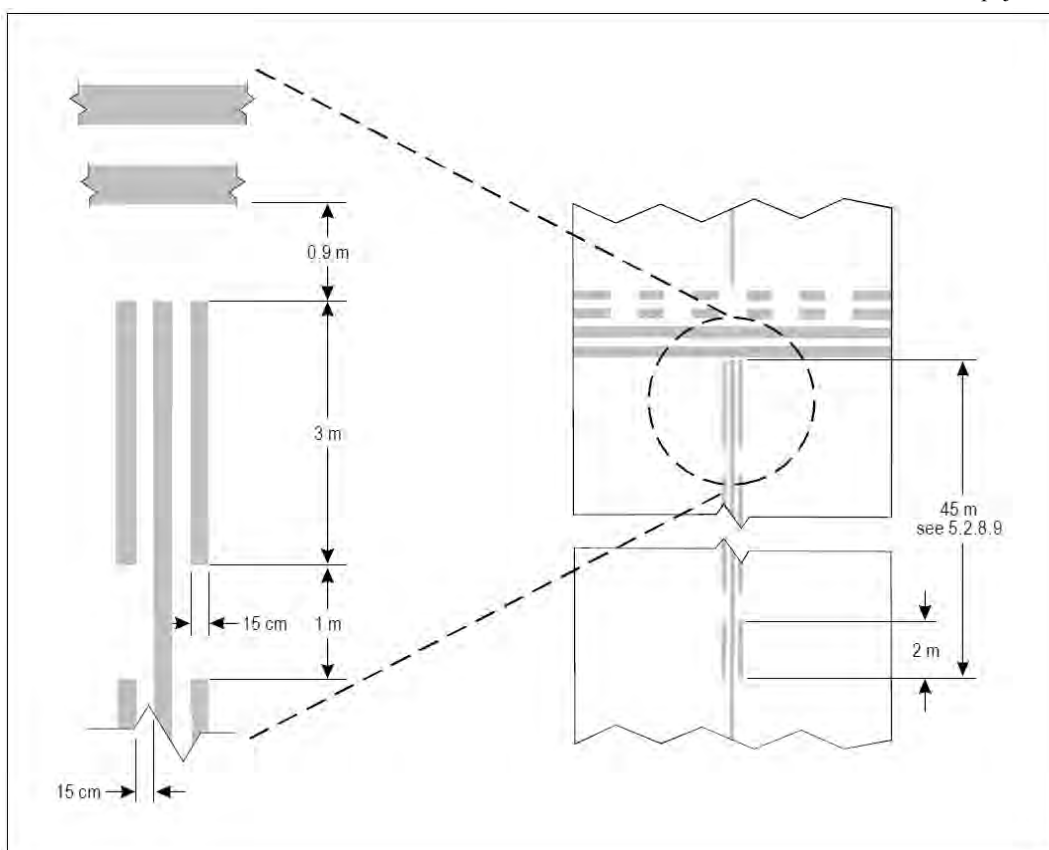
Slika 5-7. Dodatno istaknuta oznaka središnje crte staze za vožnju
