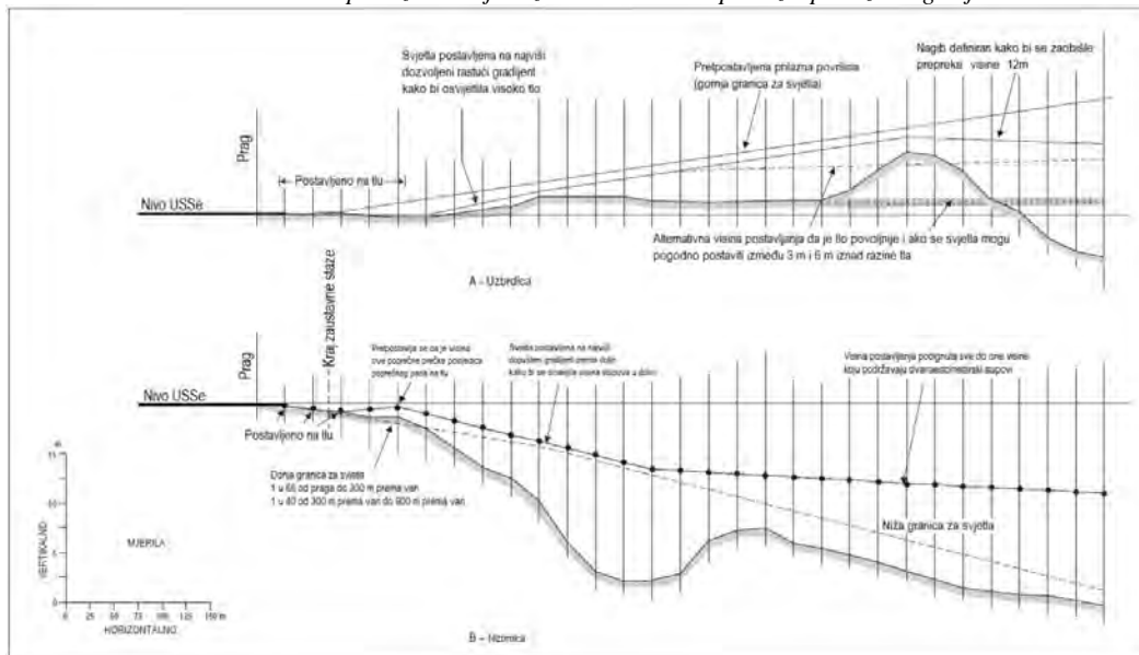
Slika A-8. Okomito dozvoljeno odstupanje instaliranja
