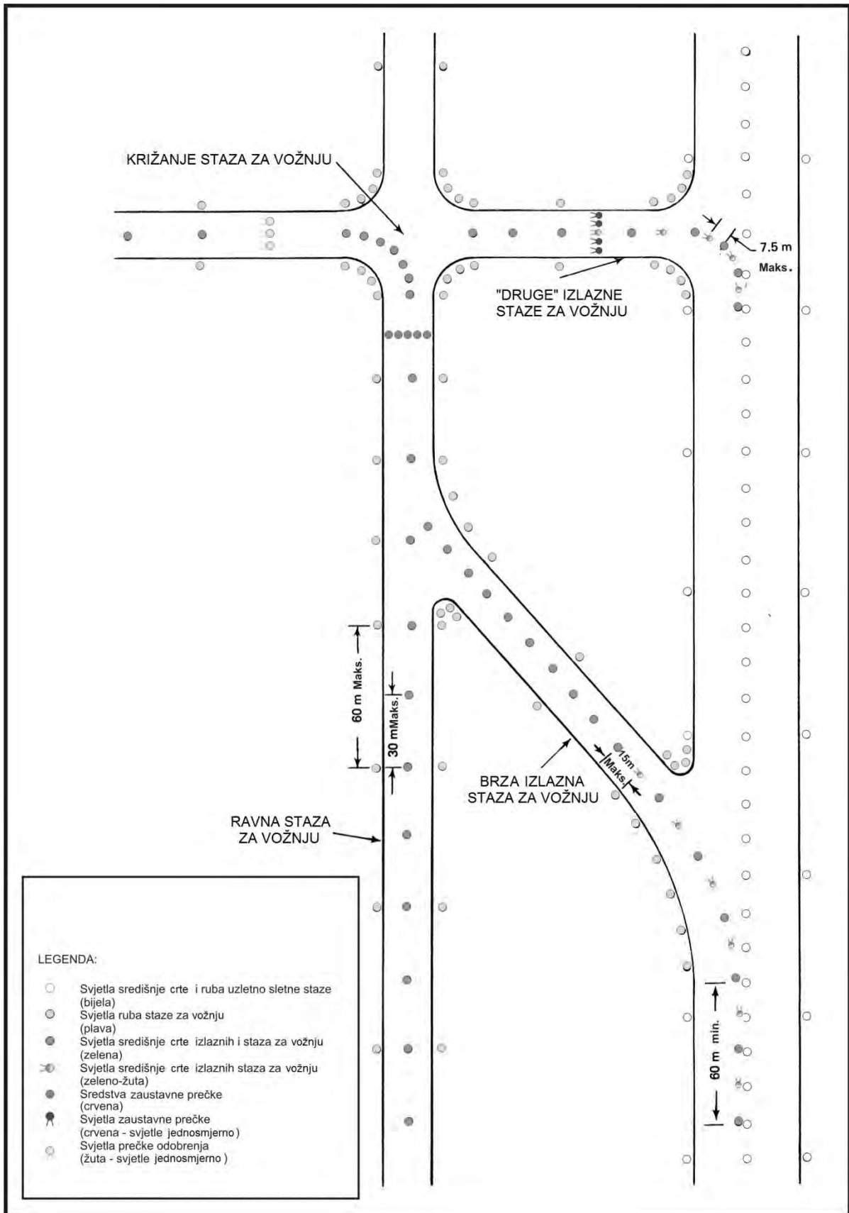
Slika 5-26 Sustavi svjetala staze za vožnju
