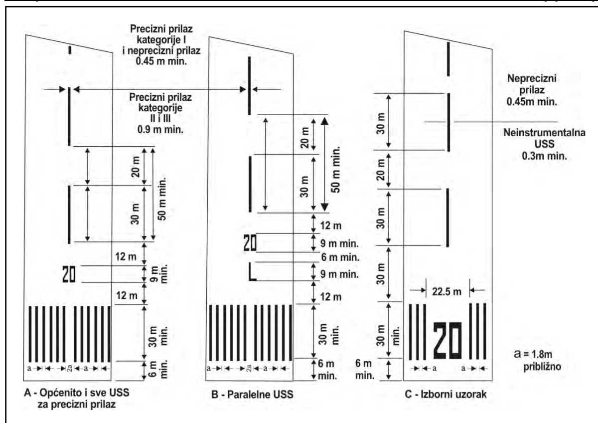
Slika 5-2. Oznake uzletno-sletne staze, središnje crte i praga
