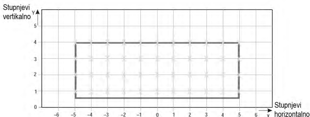
Slika A2.-21. Točke mreže koje se koriste za izračun prosječne jakosti svjetala središnje crte staze za vožnju i svjetala stop-prečke Zajedničke bilješke za slike A2.-12. do A2.-21:
