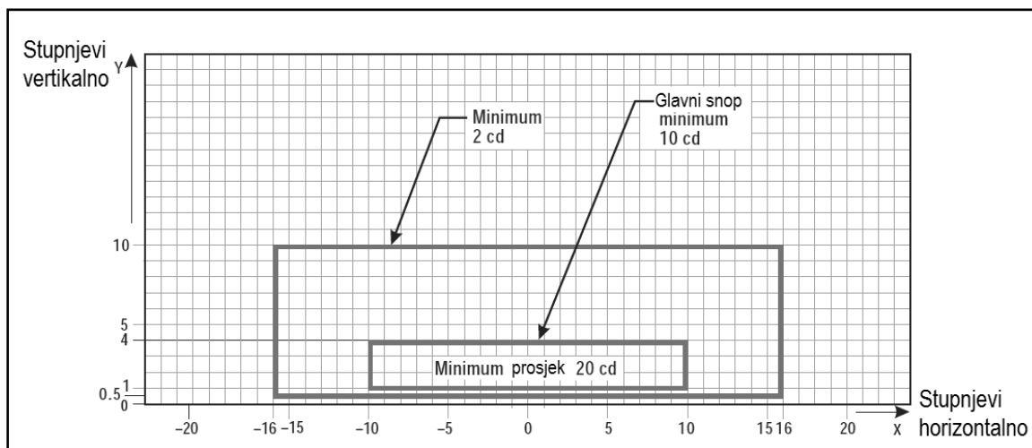
Slika A2.-14. Dijagram izokandela za svjetla središnje crte staze za vožnju (razmak 7.5 m) i svjetla stop-prečke u zakrivljenim sekcijama namijenjena korištenju u uvjetima vizualnog dometa uzletno-sletne staze vrijednosti manje od 350 m
