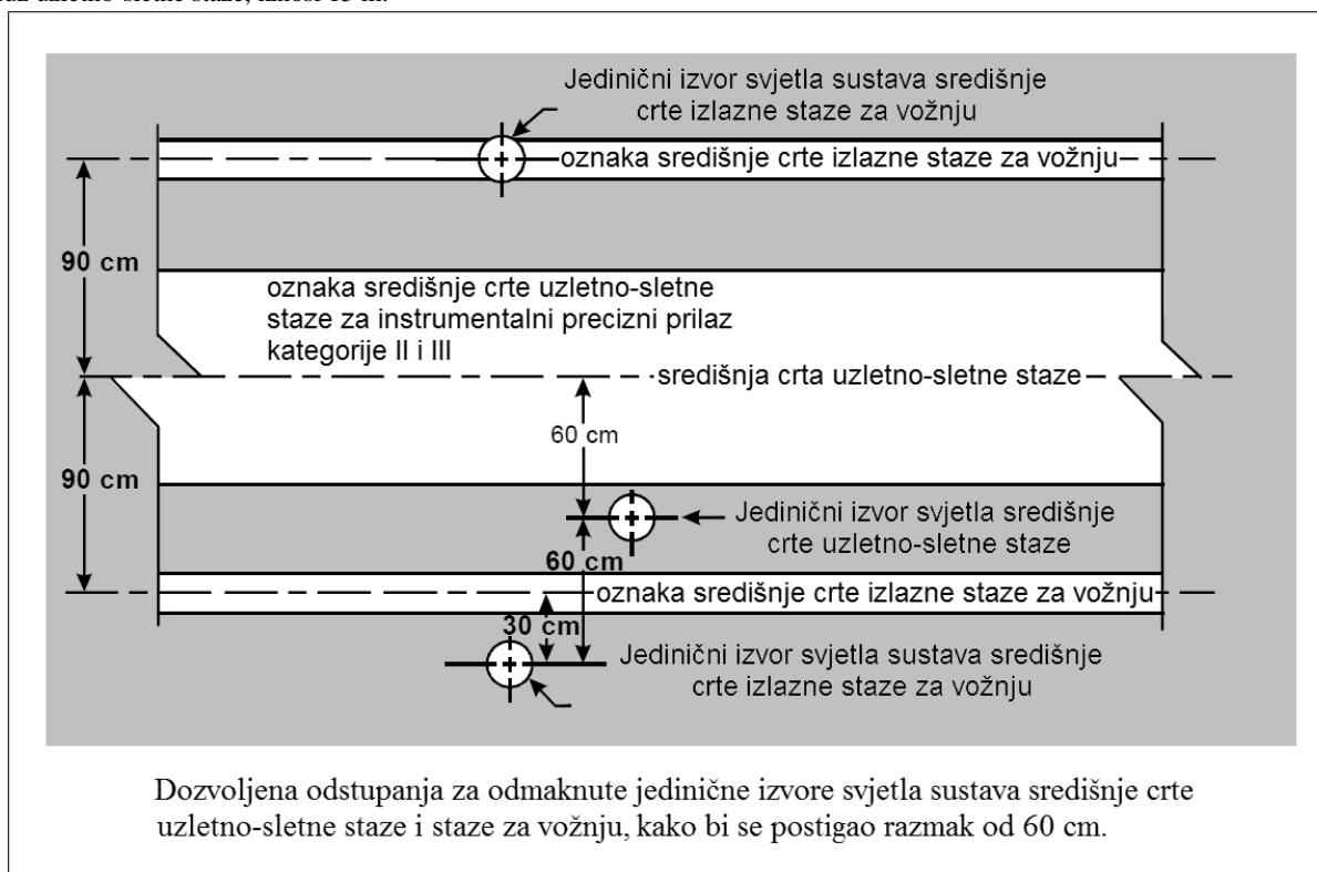
Slika 5-27. Odmaknuti jedinični izvori svjetla sustava svjetala središnje crte uzletno-sletne staze i staze za vožnju Članak 112.
