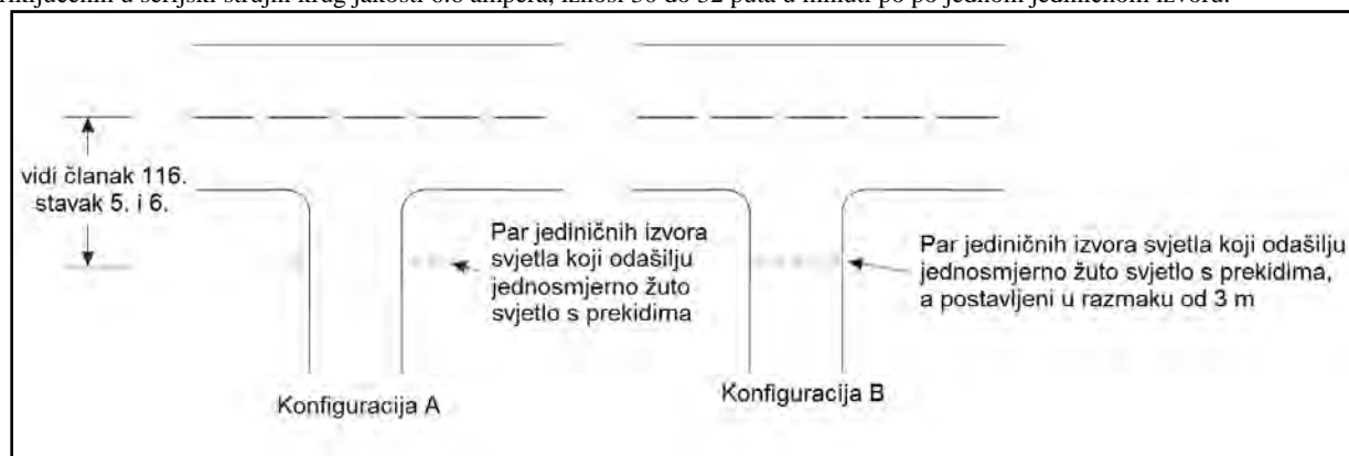
Slika 5-29. Sustav sigurnosnih svjetala uzletno-sletne staze
