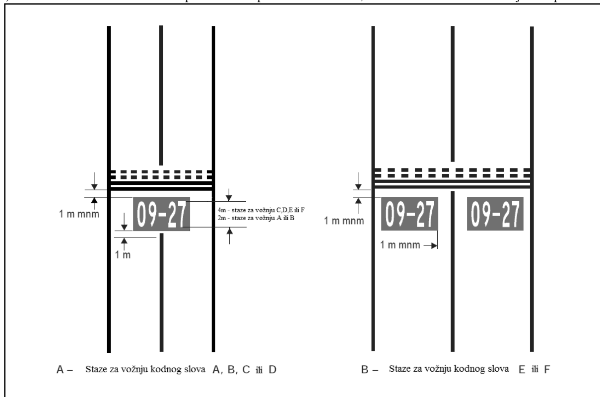
Slika 5-11. Oznake naredbi
