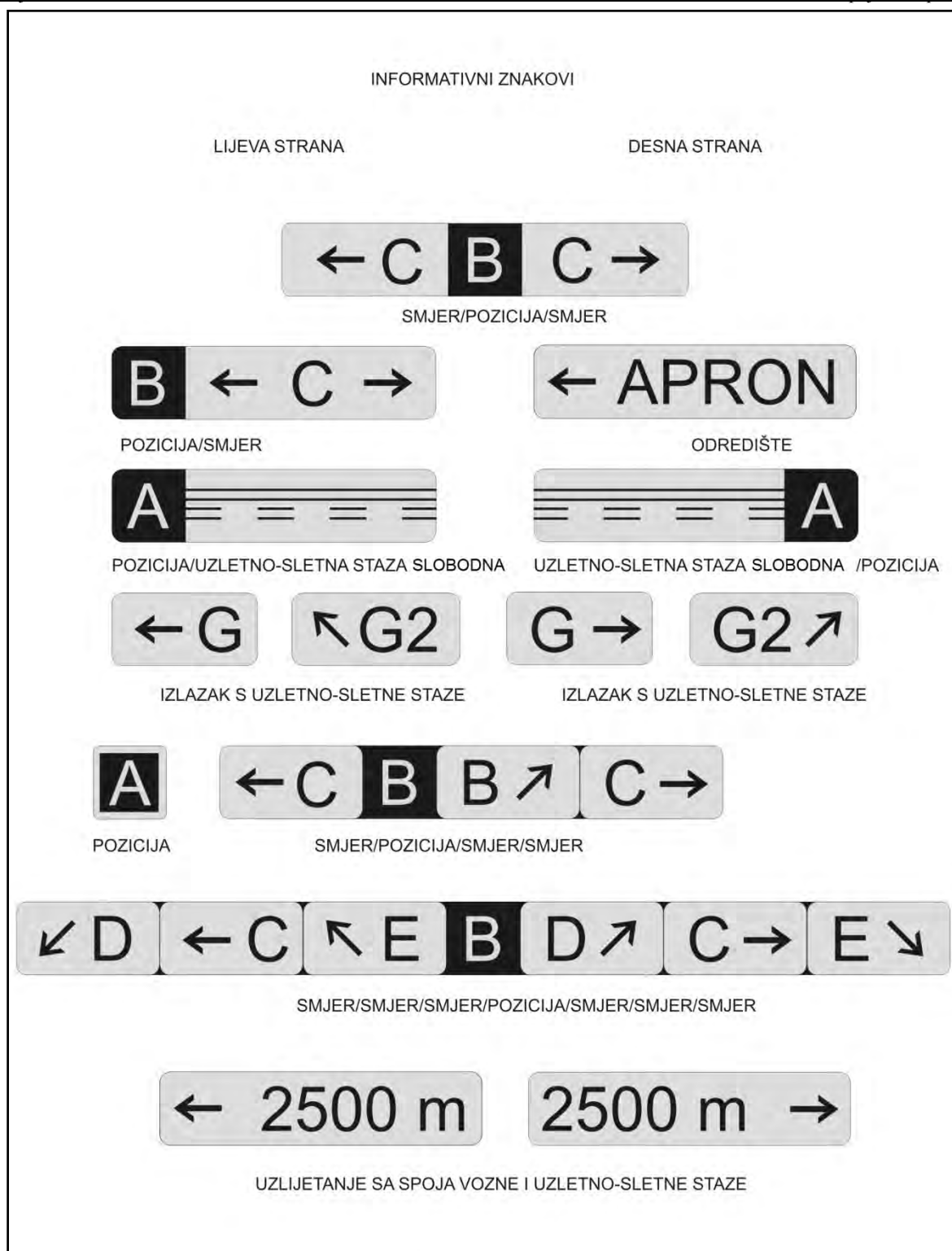
Slika 5-31. Informativni znakovi
