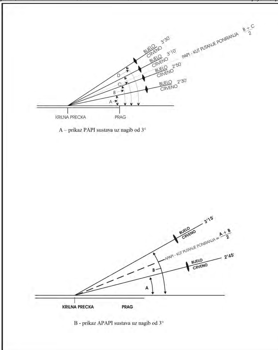
Slika 5-21 Nagib prilaza definiran za sustave PAPI i APAPI
