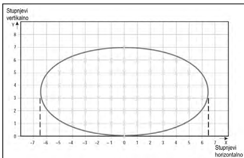
Slika A2.-11. Točke mreže koje se koriste za izračun prosječne jakosti svjetala sustava prilazne rasvjete i rasvjete uzletno-sletne staze
