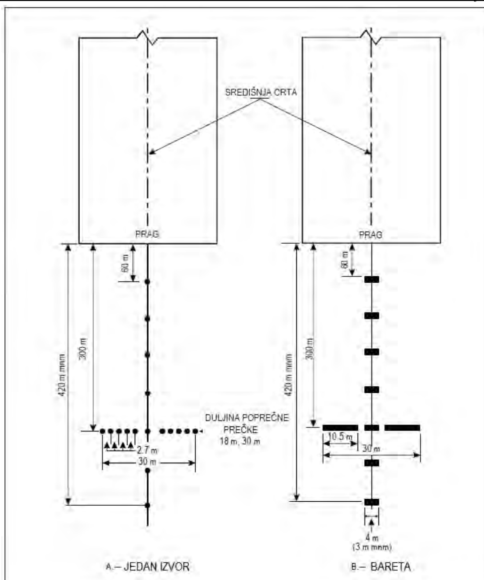
Slika A-6. Sustavi prilazne rasvjete definirani za jednostavni prilaz
