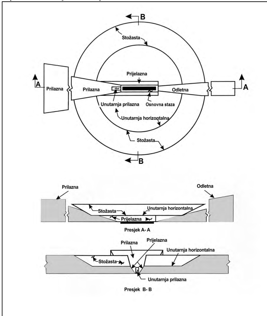
Slika 4-1 Površine ograničenja prepreka
