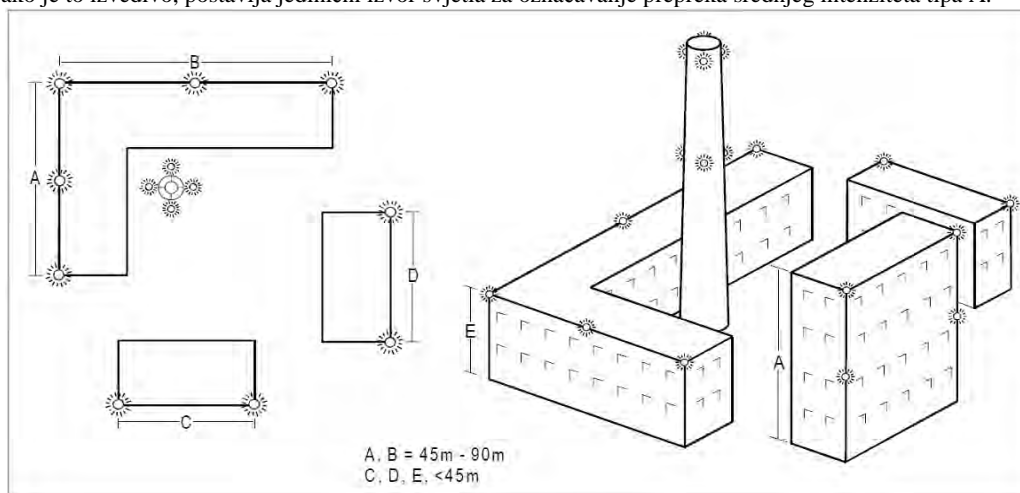
Slika 6-3. Osvjetljavanje zgrada
