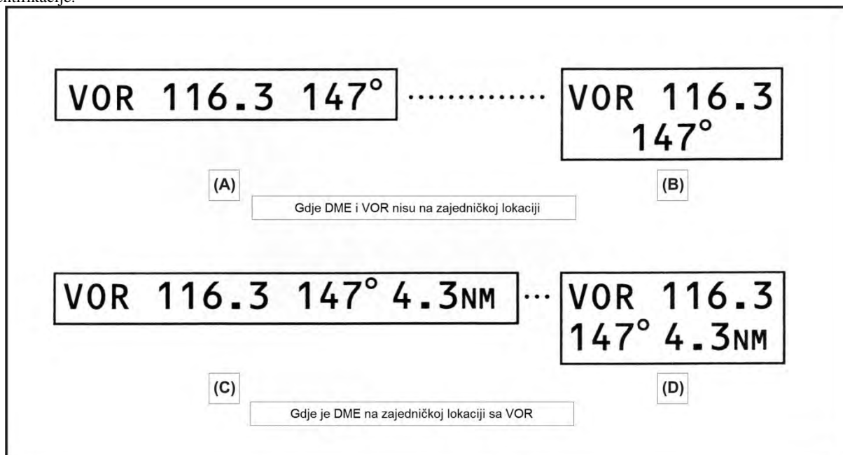
Slika 5-33. Znak VOR kontrolne točke aerodroma
