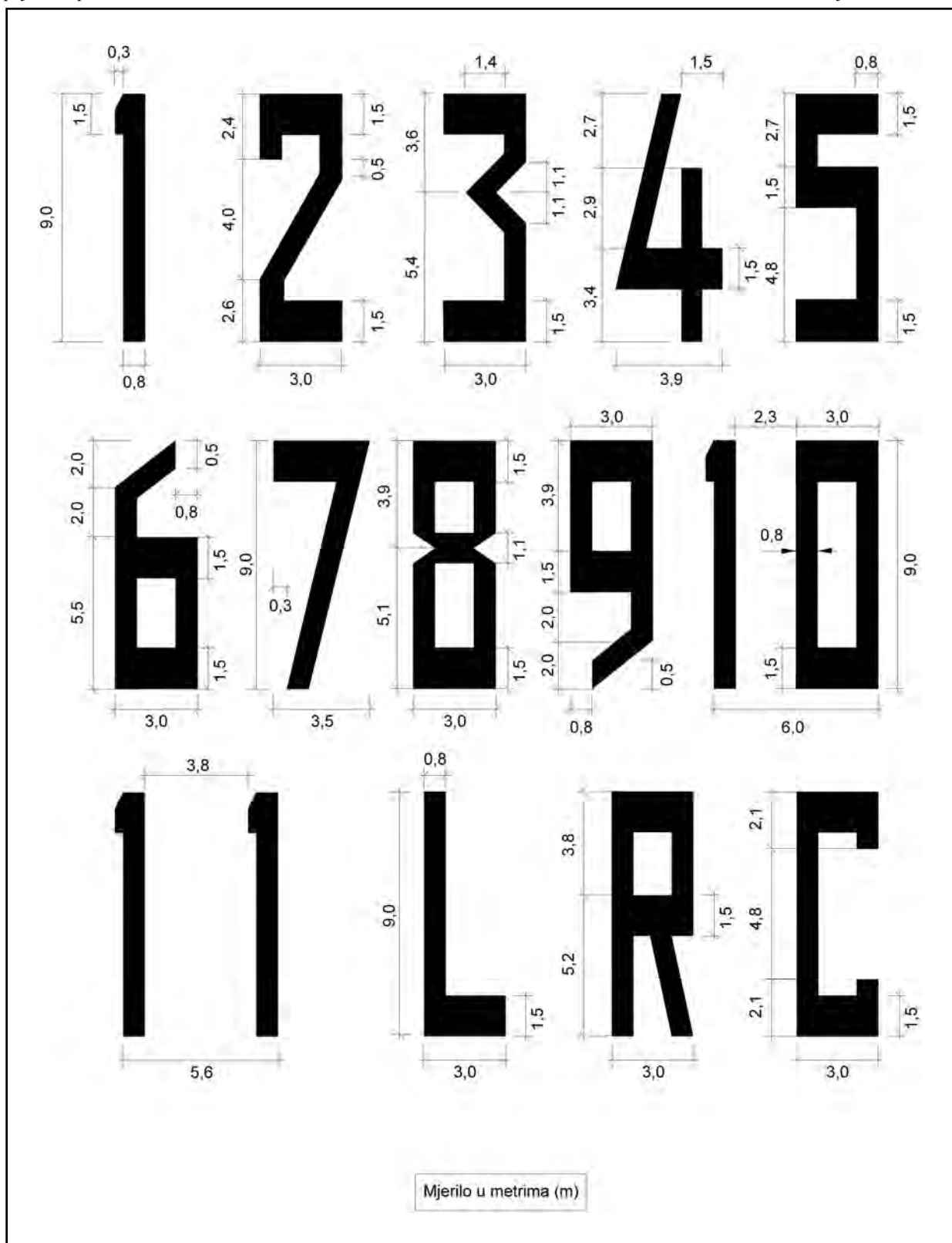
Slika 5-3. Oblik i veličina brojki i slova koji čine oznaku uzletno-sletne staze Članak 72.
