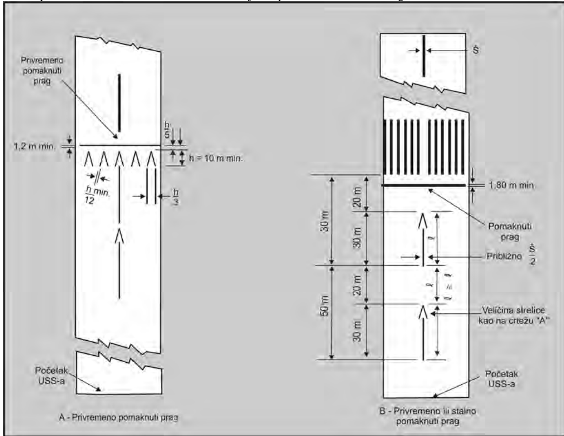
Slika 5-4. Oznake pomaknutog praga Članak 74.
