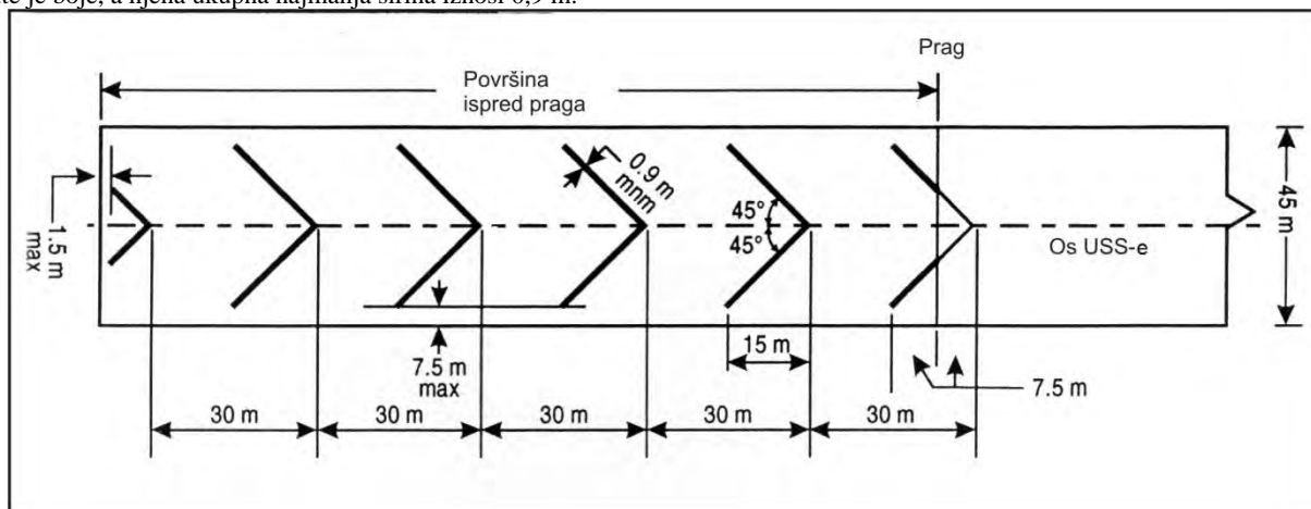
Slika 7-2. Oznaka površina ispred praga
