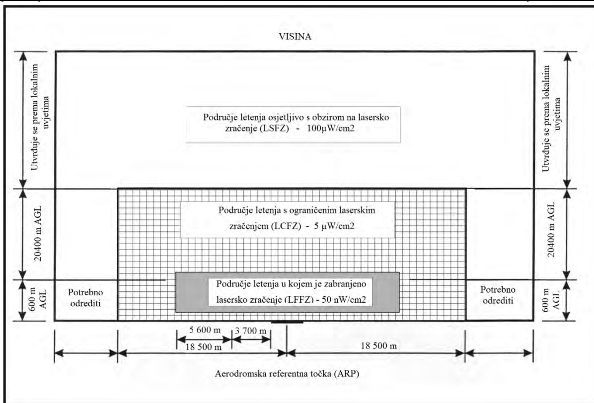
Slika 5-14. Zaštićena područja letenja s najvišim dozvoljenim vrijednostima isijavanja vidljivih laserskih zraka
