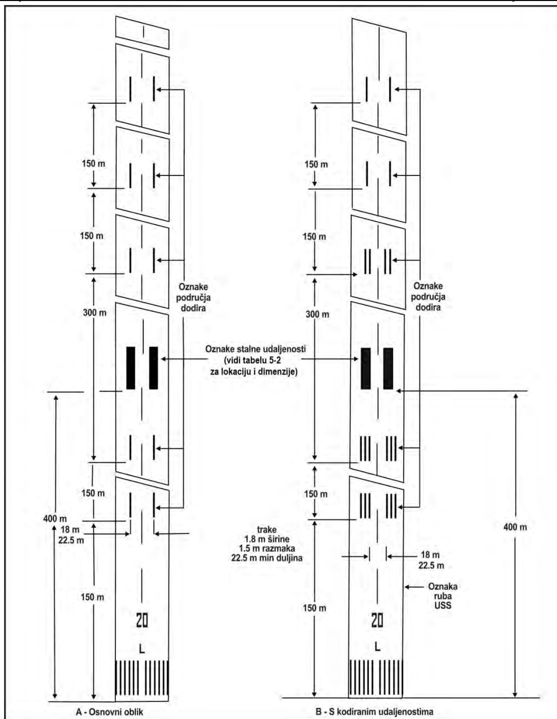
Slika 5-5. Oznake ciljne točke i područja dodira na uzletno-sletnoj stazi duljine \geq 400 m
