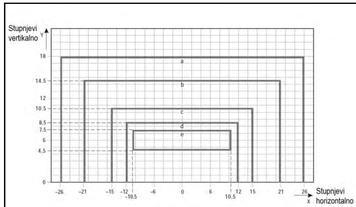
Slika A2.-16. Dijagram izokandela za svjetla središnje crte staze za vožnju (razmak 7.5 m, 15 m, 30 m) i svjetla stop-prečke u zakrivljenim sekcijama namijenjena korištenju u uvjetima vizualnog dometa uzletno-sletne staze minimalno 350 m
