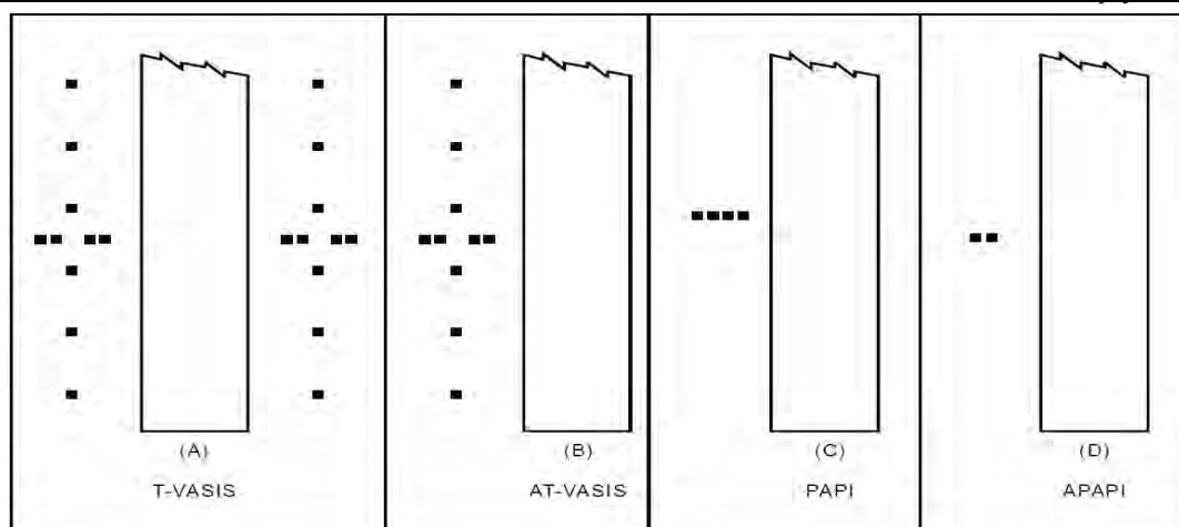
Slika 5-17. Sustavi svjetlosnih pokazivača nagiba prilaza
