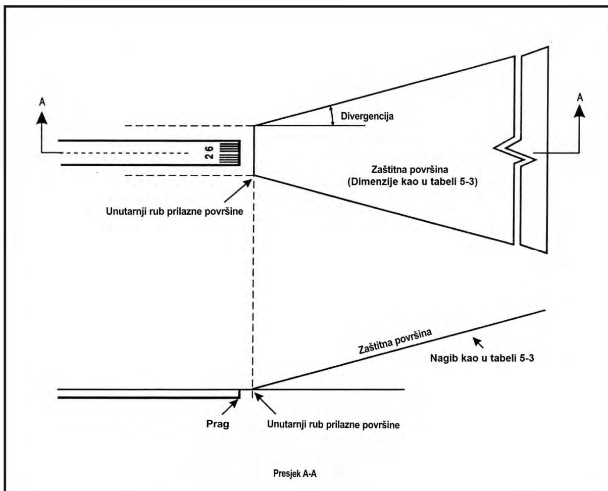
Слика 5-22. Површина слободна од препрека за системе свјетлосних показивача нагиба прилаза
