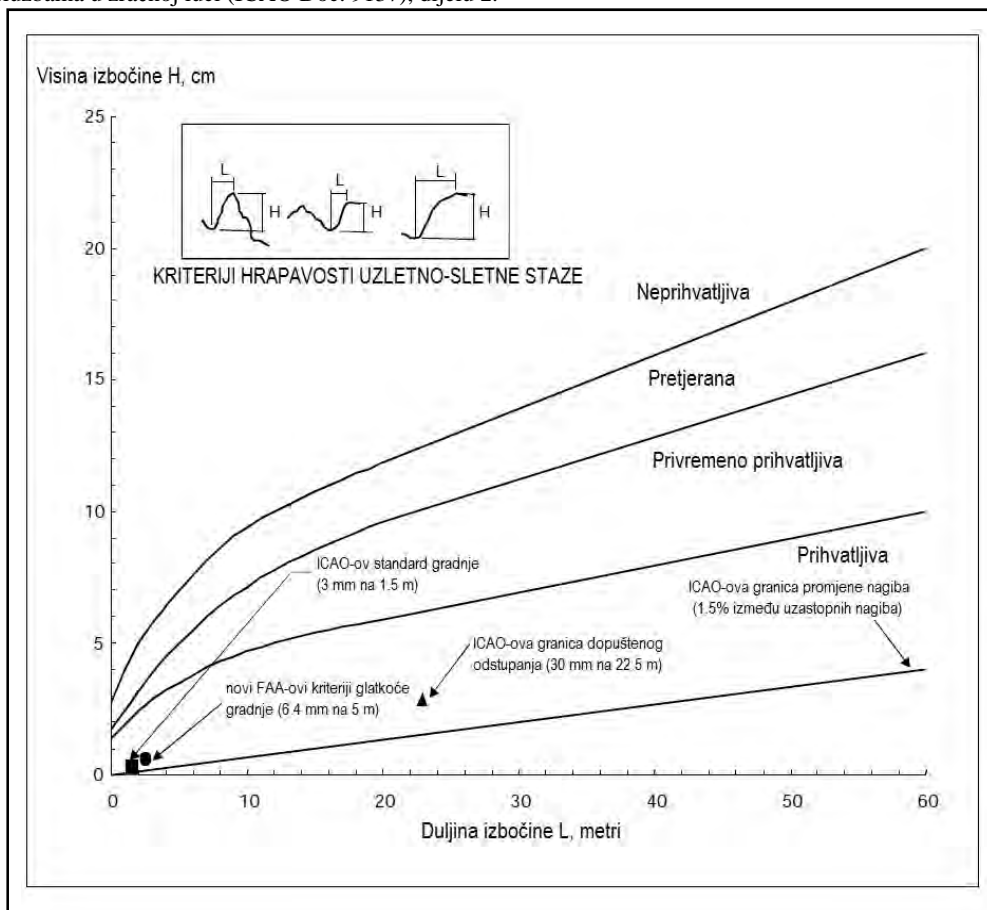
Slika A-3. Usporedba kriterija hrapavosti
