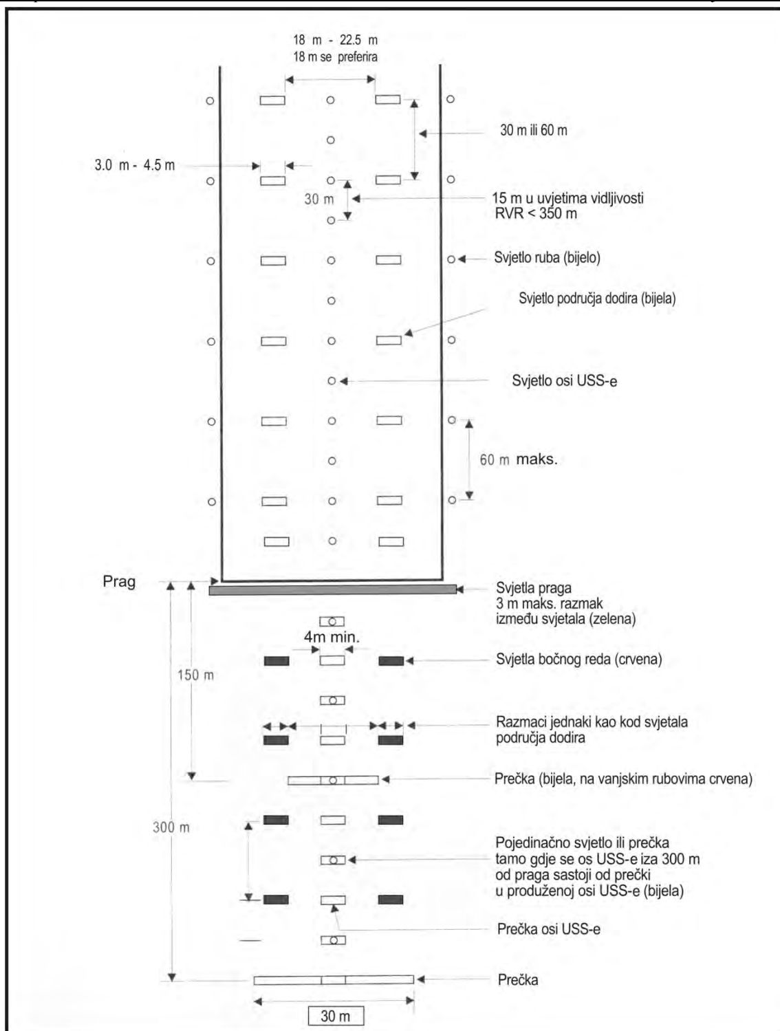
Slika 5-16. Unutarnjih 300 m sustava prilazne rasvjete i sustava rasvjete uzletno-sletne staze za instrumentalni precizni prilaz kategorije II ili III, ukoliko operator aerodroma osigura ispravnost sustava prilazne rasvjete definiran u članakku 189. stavku 8. ovog Pravilnika
