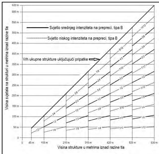
Slika A6.-2. Sustav crvenih treptajućih svjetala srednjeg intenziteta, tipa B, na preprekama
